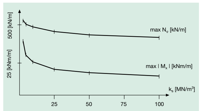
Bild 9: Maximalwerte der Schnittgrößen N_\varphi und |M_x| in Abhängigkeit vom Bettungsmodul k_s
