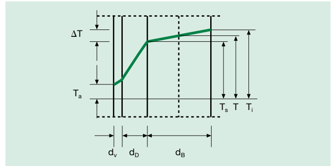
Bild 7: Temperaturprofil in der Fermenterwand
