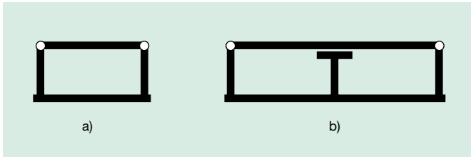
Bild 4: Fermenterabschluss mit Stahlbetonkreisplatte a) ohne Mittelstütze, b) mit Mittelstütze
