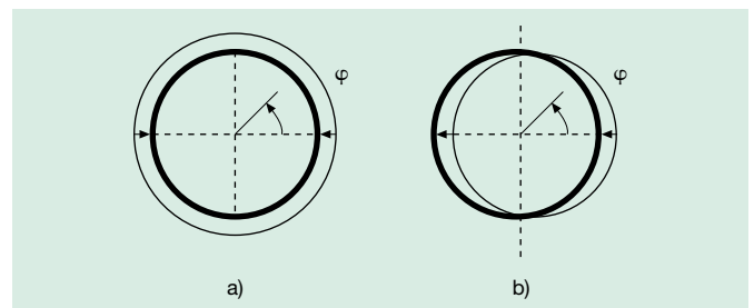
Bild 6: Verteilung der Flächenlast über Zylinderumfang a) zum Meridian \varphi = \pi / 2 symmetrisch Einwirkung ( n = 0 ) b) zum Meridian \varphi = \pi / 2 antimetrisch Einwirkung ( n = 1 )
