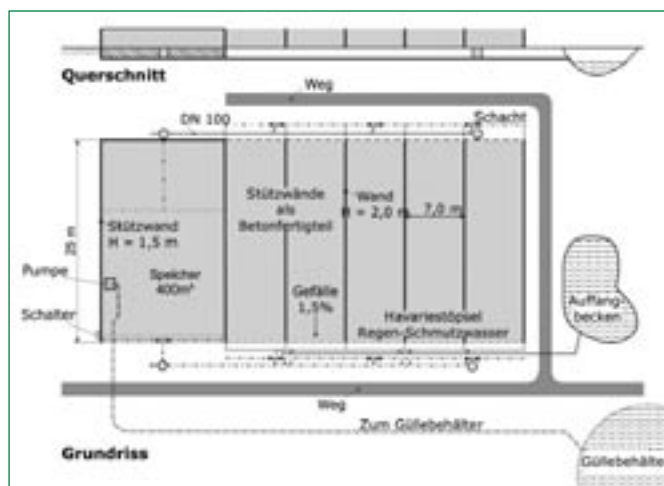
Bild 1: Grundriss und Querschnitt der neuen Festmist – Fahrsilo – Kombination aus Stahlbeton
