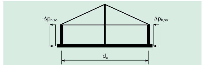
Bild 5: Seismische Einwirkung nach DIN 1055-6, antimetrische Flächenlast mit \Delta p_{h,so} = \gamma \cdot a / g \cdot d_c / 2 (a: horizontale Erdbeschleunigung)
