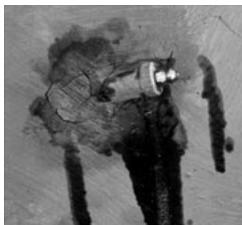
Bild 2: Eingebohrte Verpressdüse für Injektion zur Betoninstandsetzung
