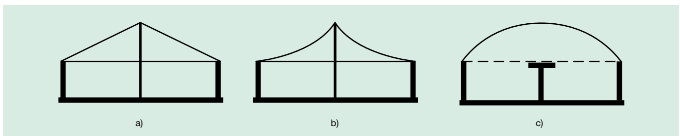
Bild 3: Fermenterabschluss mit Hüllkonstruktion, a) Kegelfläche, b) Sattelfläche, c) Kugelfläche
