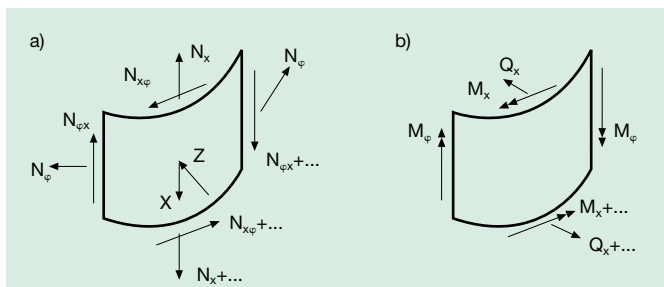
Bild 8: Flächenlasten X und Z und Schnittgrößen in der Behälterwand a) Membranspannungszustand, b) Biegespannungszustand
